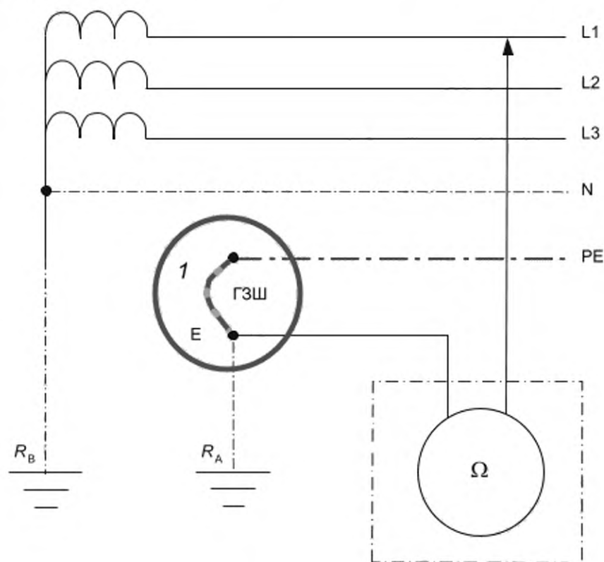
Рисунок С.2 — Измерение активного сопротивления заземлителя с применением прибора измерения полного сопротивления петли замыкания на землю
