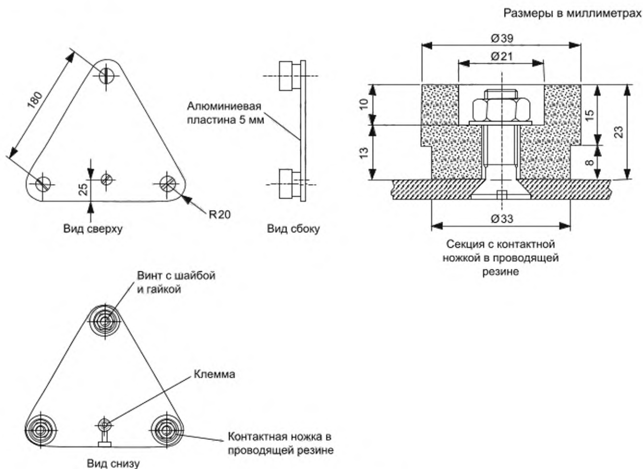
Рисунок В.1 — Испытательный электрод 1
